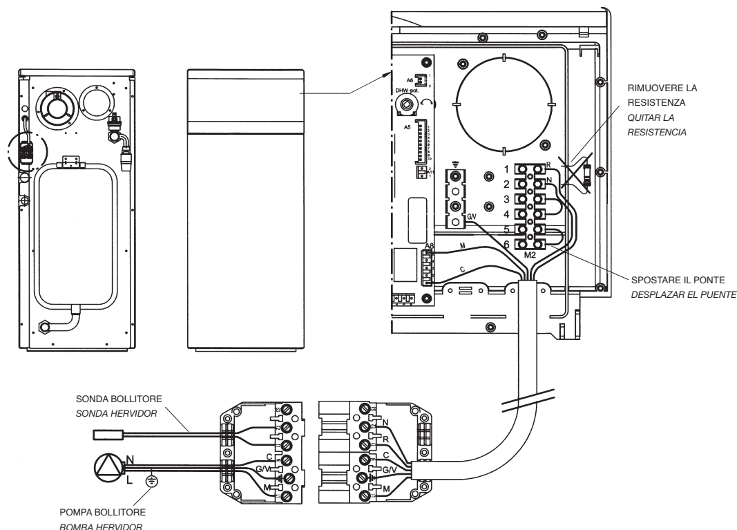
Figura 6: Connessione elettrica cavo alimentazione - sonda sanitario Figura 6: Conexión eléctrica cable de alimentación - sonda sanitario
