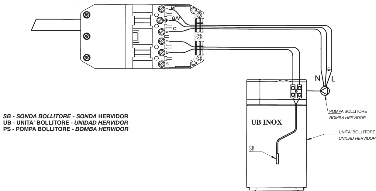
Figura 8: Connessione elettrica con Unità bollitore BAXI SLIM UB INOX Figura 8: Conexión eléctrica con Unidad hervidor BAXI SLIM UB INOX
